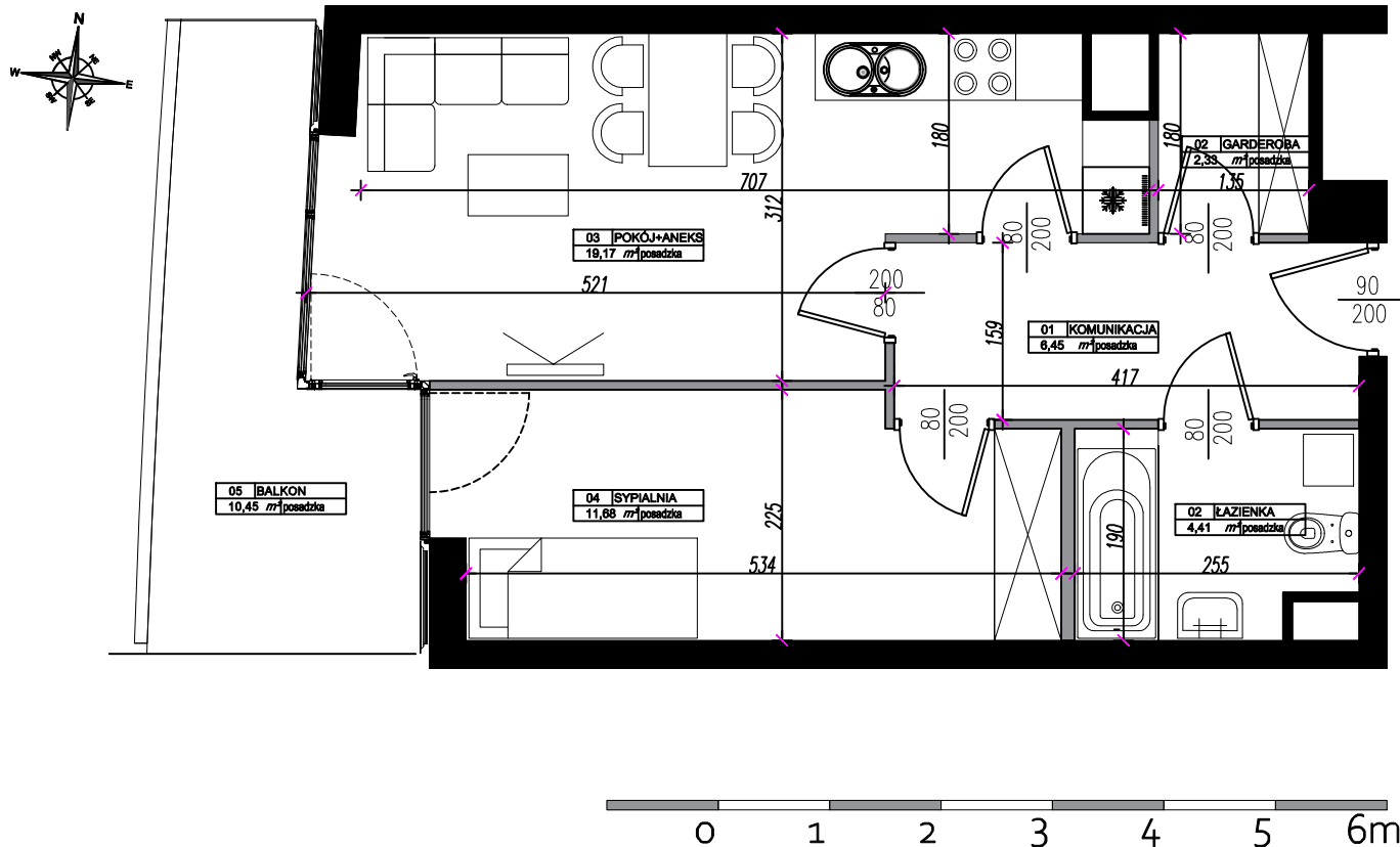
RZUT MIESZKANIA:
