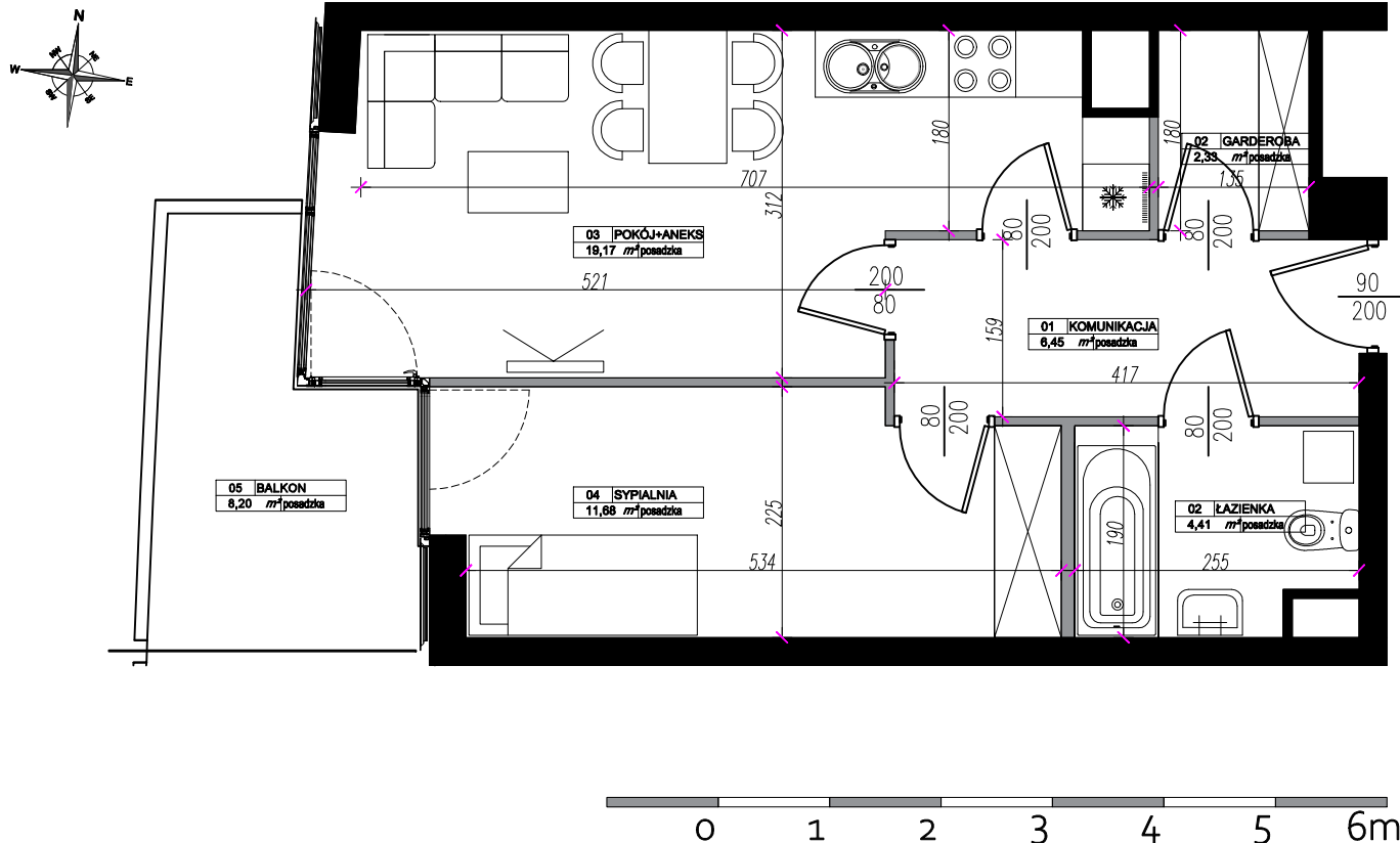
RZUT MIESZKANIA:
